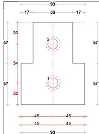
Tussenneut 90mm Sponning Bi 57mm Art. nr. 464417
