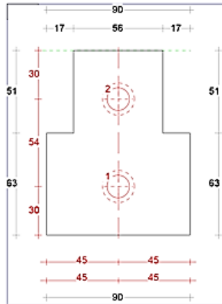
Tussen neut 90mm Sponning Bi 51mm Art. nr. 464415
