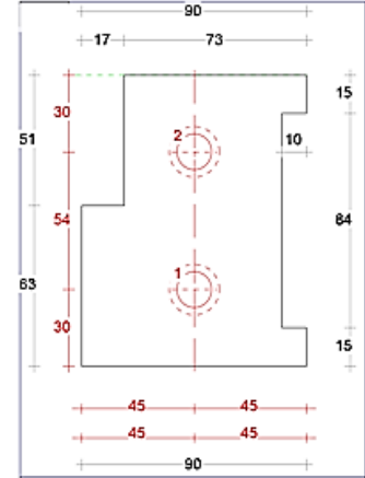
Neut rechts 90mm Sponning Bi 51mm Art. nr. 464433
