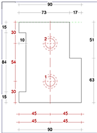
Neut links 90mm Sponning Bi 51mm Art. nr. 464432
