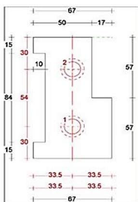
Wisselneut links 67mm Sponning Bi 57mm Art. nr. 464560
