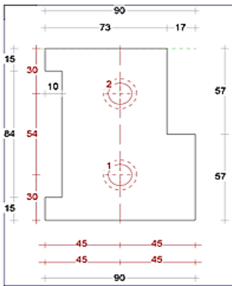
Neut links 90mm Sponning Bi 57mm Art. nr. 464434
