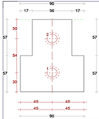
Tussen neut 90mm Sponning Bi 57mm Art. nr. 464417
