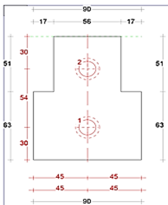
Tusseneut 90mm Sponning Bi 51mm Art. nr. 464415
