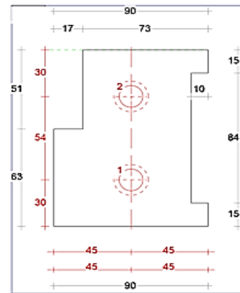
Neut rechts 90mm Sponning Bi 51mm Art. nr. 464433
