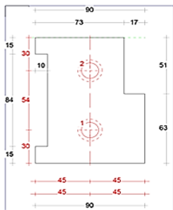
Neut links 90mm Sponning Bi 51mm Art. nr. 464432
