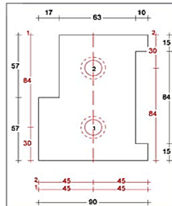
Wisselneut rechts 90mm Sponning Bi 57mm Art. nr. 464564
