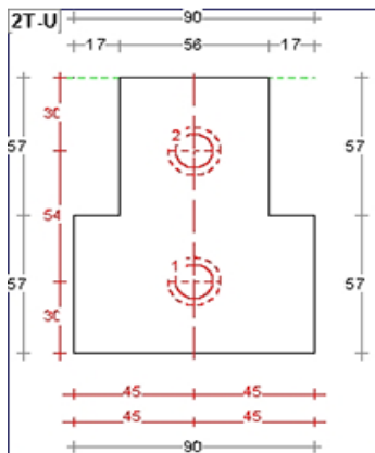
Wisseltussenneut 90mm Sponningen Bi 57mm Art. nr. 464569
