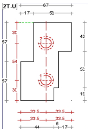
Wisseltussenneut 67mm Sponning Bu 72mm / Bi 57mm Art. nr. 464561
