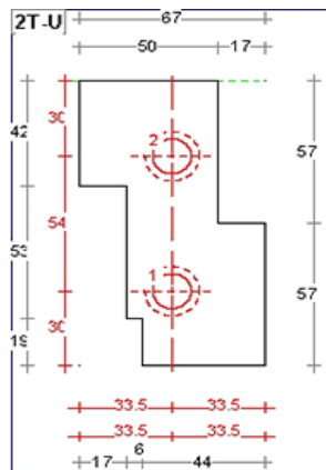
Wisseltussenneut 67mm Sponning Bu 72mm / Bi 57mm Art. nr. 464563
