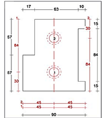
Wisselneut rechts 90mm Sponning Bi 57mm Art. nr. 464476
