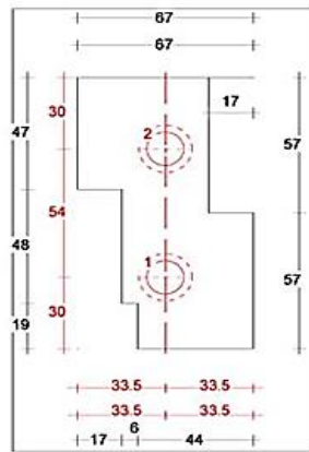
Wisseltussenneut 67mm Sponning Bu 67mm / Bi 57mm Art. nr. 464473
