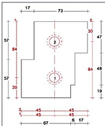
Wisseltussenneut 90mm Sponning Bu 67mm / Bi 57mm Art. nr. 464475
