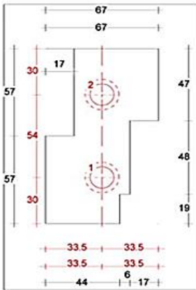
Wisseltussenneut 67mm Sponning Bu 67mm / Bi 57mm Art. nr. 464471
