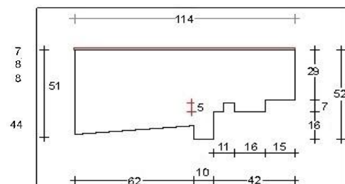
Neut contraprofiel
