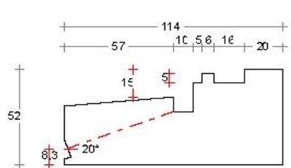
Dorpel Bu 52 x 114mm Sponning Bu 67mm Art. nr. 4644051
