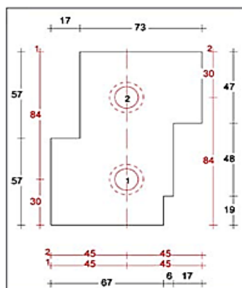
Wisseltussenneut 90mm Sponning Bu 67mm / Bi 57mm Art. nr. 464475
