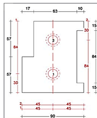
Wisselneut rechts 90mm Sponning Bi 57mm Art. nr. 464476
