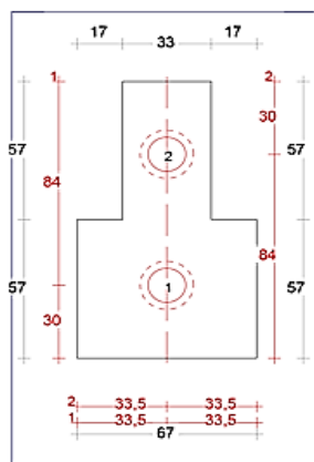
Wisseltussenneut 67mm Sponningen Bi 57mm Art. nr. 464479
