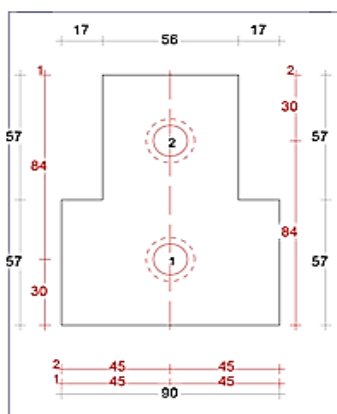
Wisseltussenneut 90mm Sponningen Bi 57mm Art. nr. 464480
