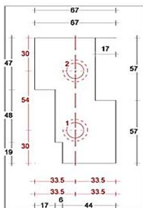
Wisseltussenneut 67mm Sponning Bu 67mm / Bi 57mm Art. nr. 464473
