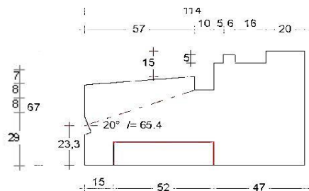
Dorpel Bu 67 x 114mm Sponning Bu 67mm Art. nr. 464405 zonder loodspinning Art. nr. 4644055 met loodspinning
