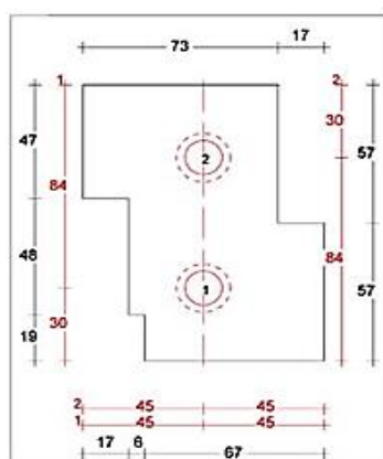
Wisseltussenneut 90mm Sponning Bu 67mm / Bi 57mm Art. nr. 464477
