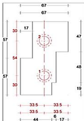
Wisseltussenneut 67mm Sponning Bu 67mm / Bi 57mm Art. nr. 464471
