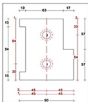
Wisselneut links 90mm Sponning Bi 57mm Art. nr. 464474
