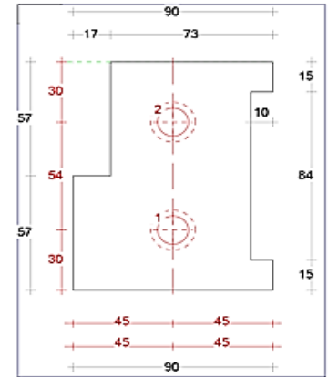
Tussenneut 90mm Sponning Bi 57mm Art. nr. 464417
